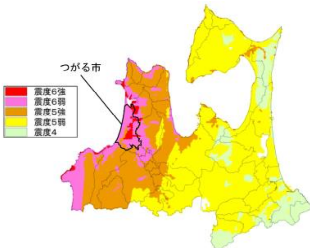
図 2-1 日本海側海溝型地震による震度分布
