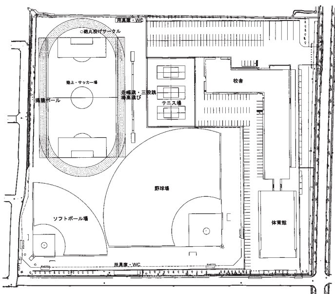
【木造中学校グラウンド整備工事 全体配置図】
