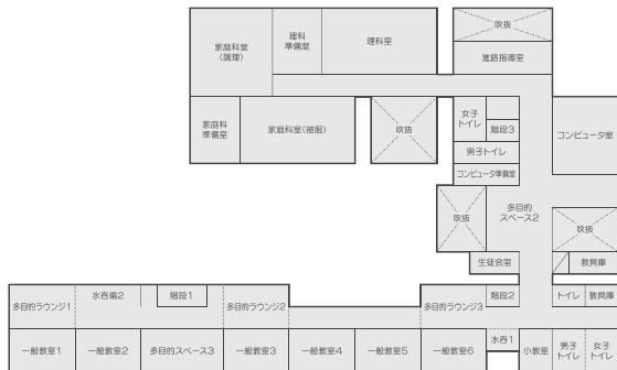
2F 校舎平面図
