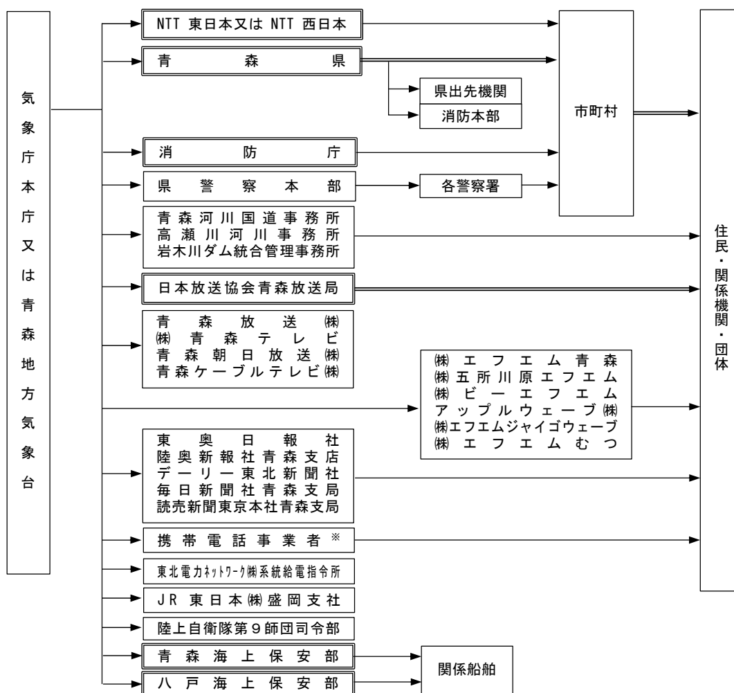
気象予報・警報・情報伝達系統図
