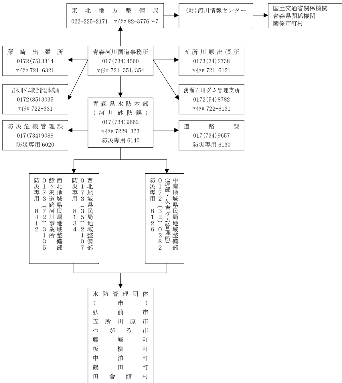
岩木川水防警報伝達系統図（岩木川、平川、浅瀬石川、旧大峰川、土淵川）
